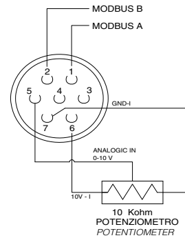
CONNETTORE SEGNALE I/O CONNECTOR
